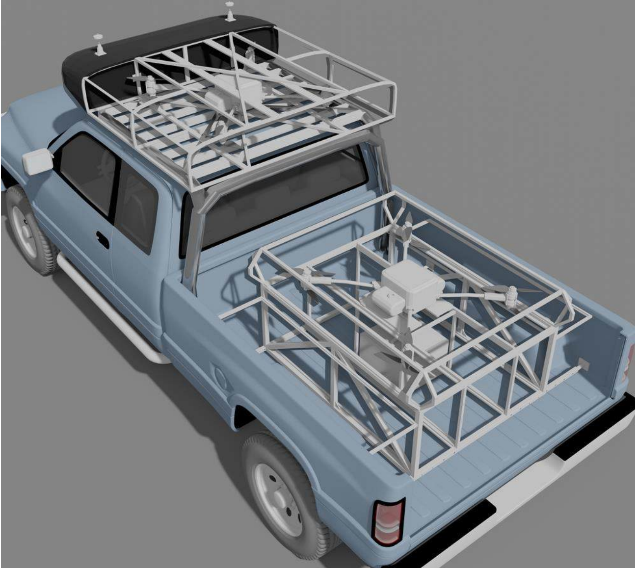
Рис. 2. Дизайн системи для запуску транспортних дронів з автомобіля (показано без захисних кожухів)
