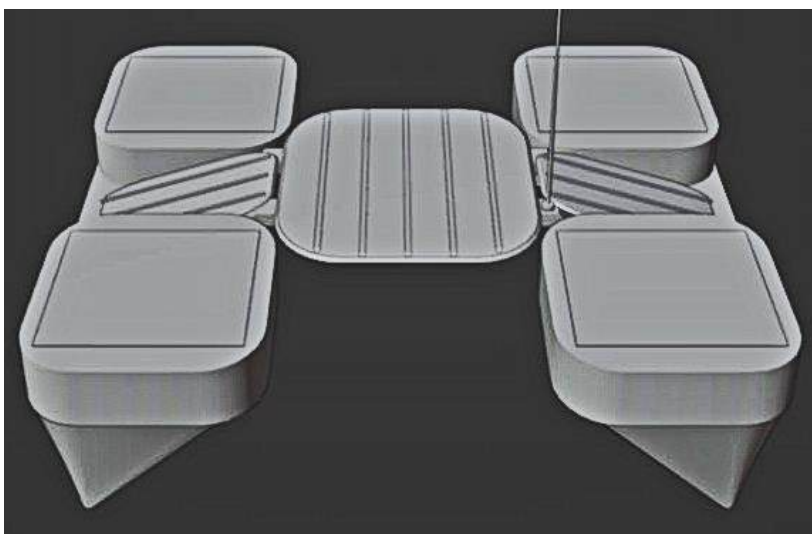
Рис. 2. Дизайн-концепція станції для підзарядки дронів на основі катамаранної конструкції
