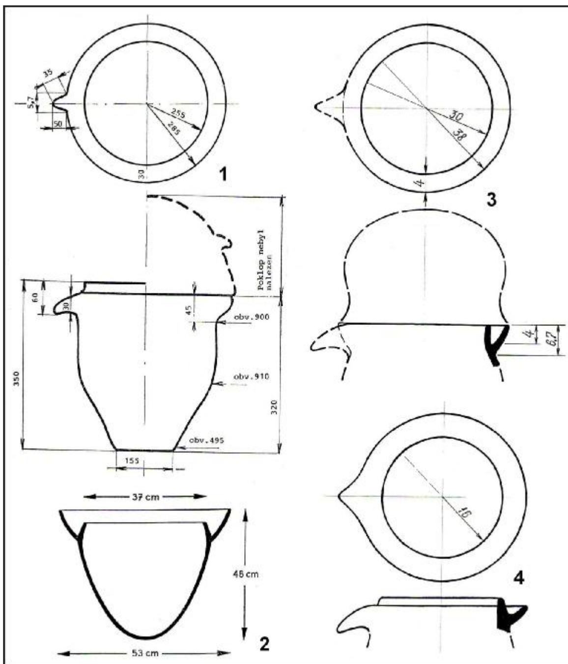
Рис. 3. Схеми та метричні параметри знахідок зі Спішського Штвртоку (1), Тепе Гаура (2) [42], Коновки (3) та Поливаного Яру (4).
