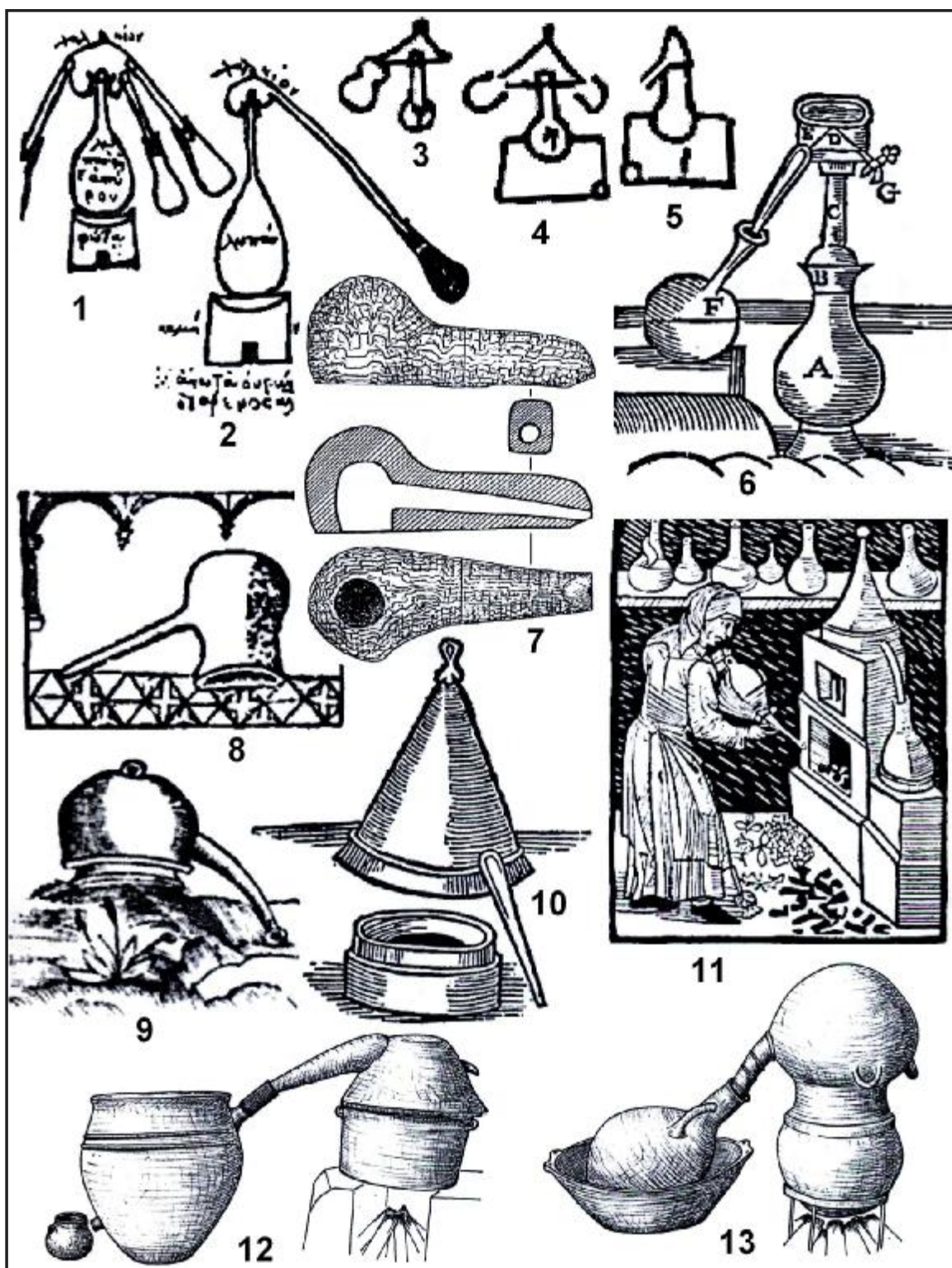
Рис. 6. Зарисовки (1-6, 8-11) та археологічні знахідки (7, 12-13) дистиляторів: 1-2 – прилади олександрійських хіміків; 3-5 – схеми апаратів з арабських манускриптів; 6, 8-11 – європейські аламбіки різних модифікацій ранньонового часу; 7 – перехідник-охолоджувач з Берестечка; 12-13 – дистиляційні апарати з Піргоса [29; 25; 20; 27].
