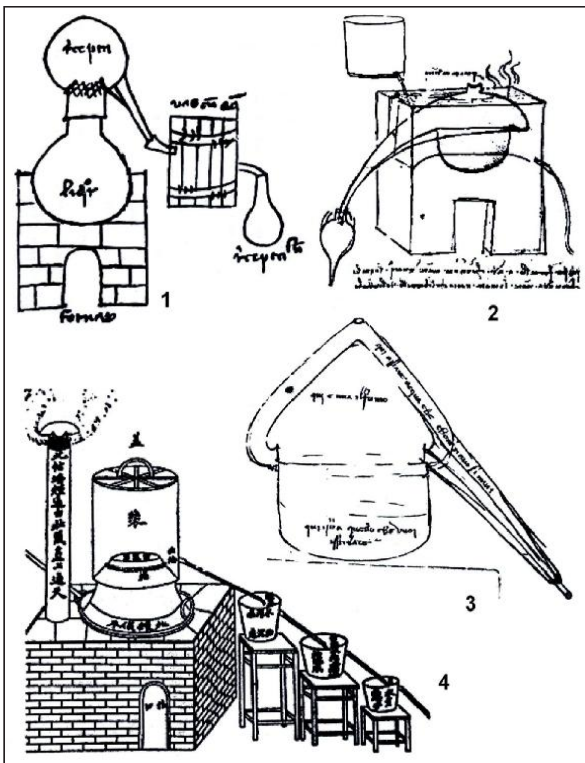
Рис. 4. Схеми дистиляційних апаратів з Європи (1-3) та Китаю (4) [29; 25].
