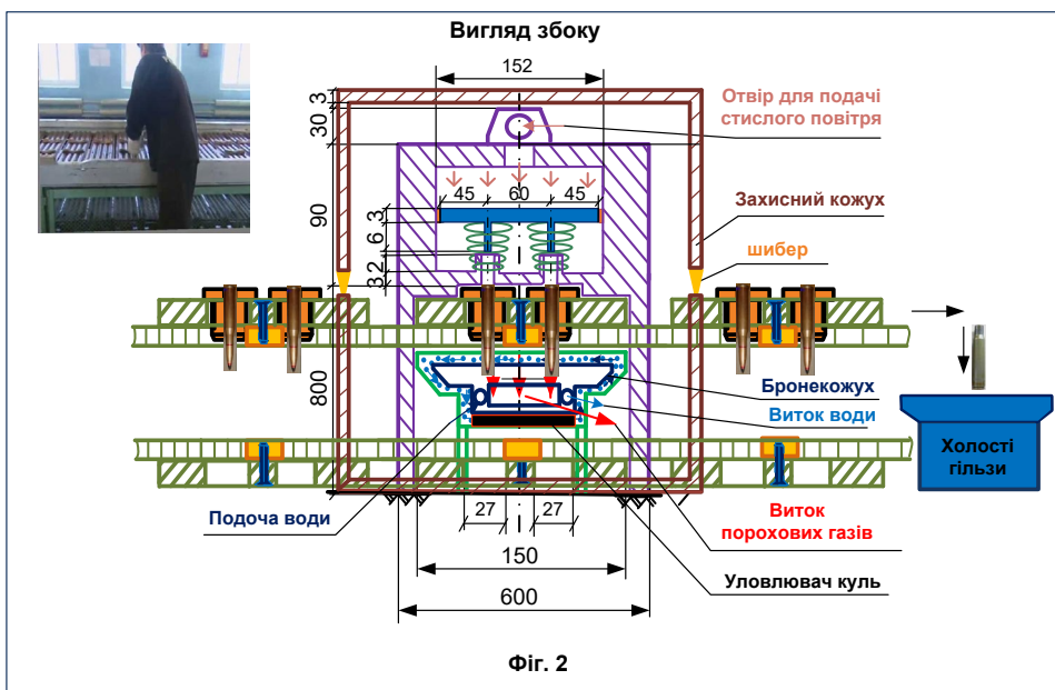
Рисунок 2. Установка для розрядження 5,45–14,5-мм НСЗ
