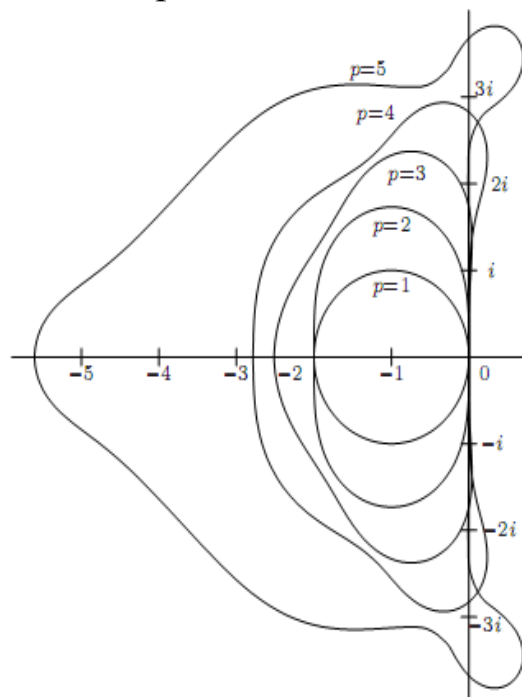
Рис. 12.7. Області стійкості методів Рунге–Кутти порядку 1-5
