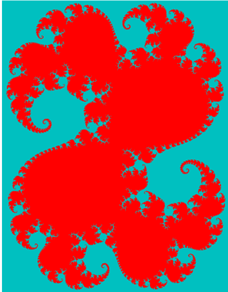
Рис. 6.4. Множина Жюліа
