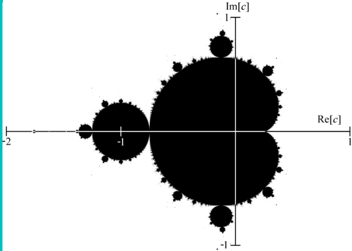
Рис. 6.5. Множина Мандельброта
