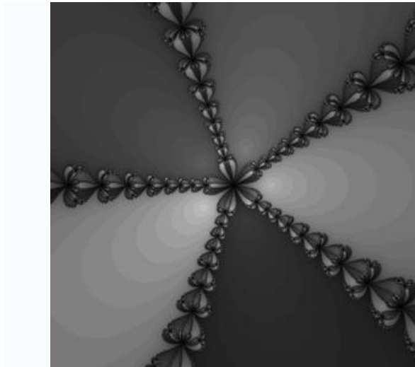
Рис. 6.6. Басейни Ньютона. Областям темнішого кольору відповідають початкові значення з більшою кількістю ітерацій
