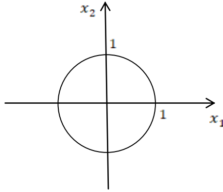
Рис. 3.3. \|x\|_2 = 1
