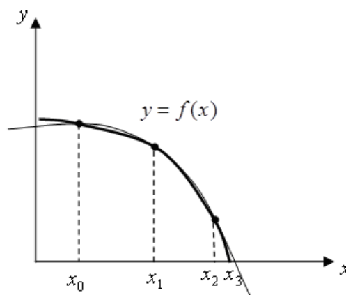
Рис. 6.3. Метод парабол
