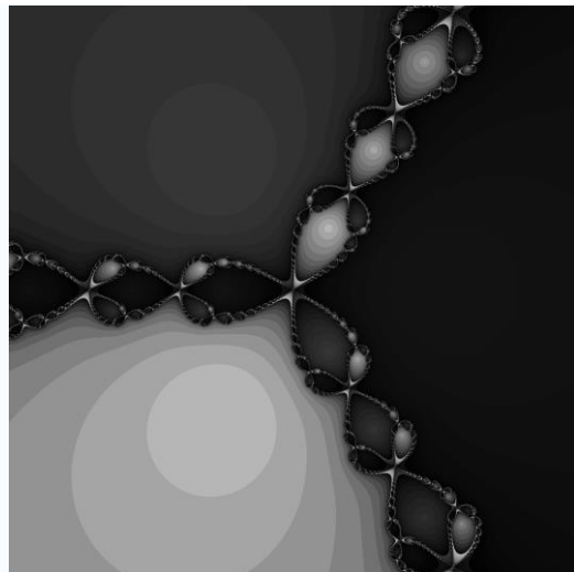
Рис. 6.6. Басейни Ньютона. Областям темнішого кольору відповідають початкові значення з більшою кількістю ітерацій
