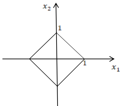
Рис. 3.1. \|x\|_1 = 1
