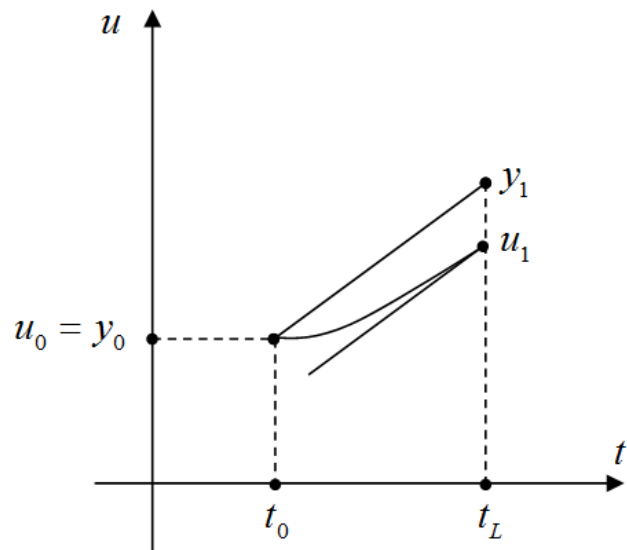
Рис. 12.2. Неявний метод Ейлера
