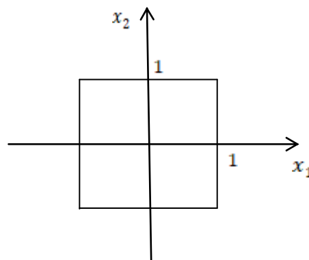
Рис. 3.2. \|x\|_\infty = 1
