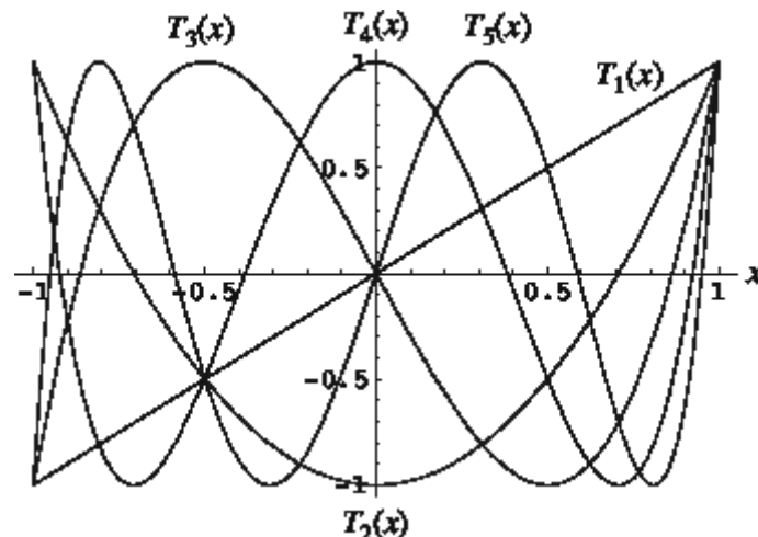
Рис. 4.1. Графіки многочленів Чебишева T_n(x) , n = \overline{1, 5}
