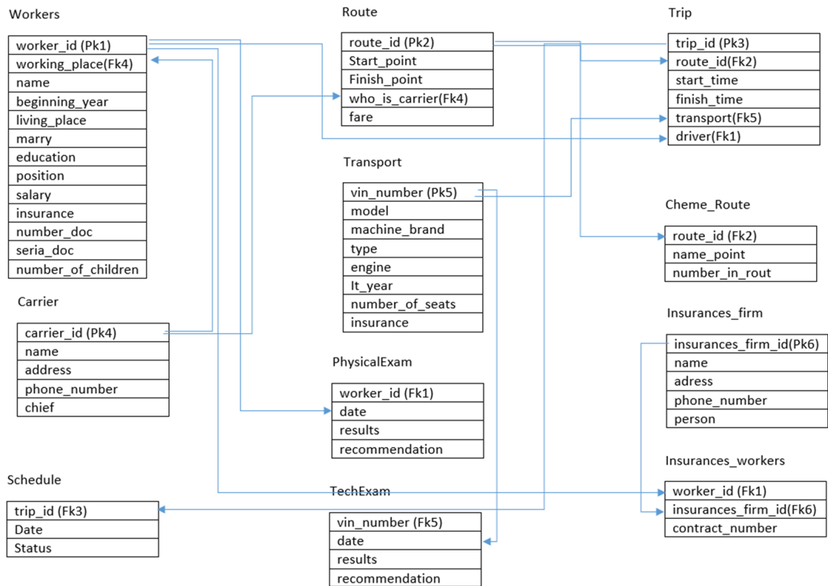
Схема БД.
