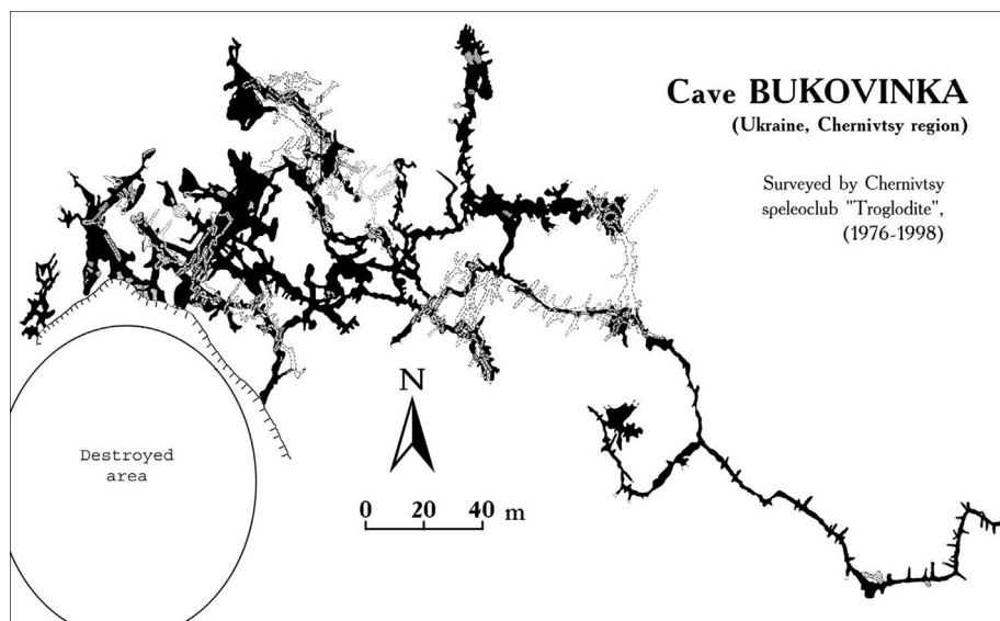
Рис. 2. План печери Буковинка (за Bondar, Ridush 2015)
