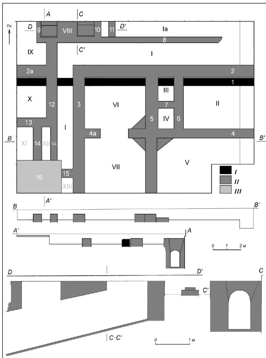
Рис. 2. План і профілі мурувань південної частини мечеті за результатами досліджень 2019 р.
