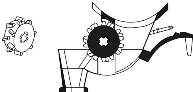
Рисунок. 2. Шевронна катушка висівного апарату сівалки Bertini.
