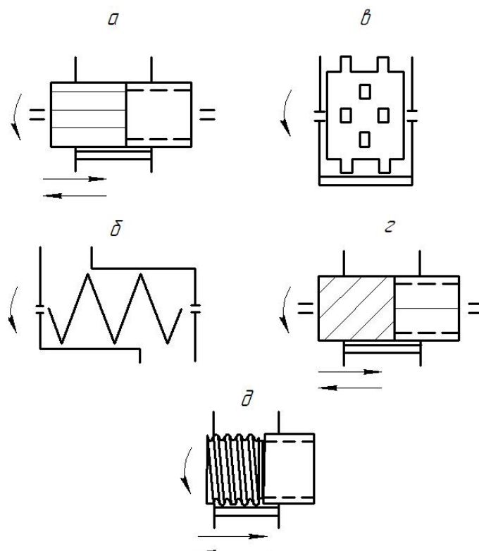
Рисунок. 4. Схеми висівних апаратів: а - жолобковий катушковий; б - шнековий; в - штифтовий; г - катушковий з жолобками, розташованими по гвинтовій лінії; д - катушковий гвинтовий.
