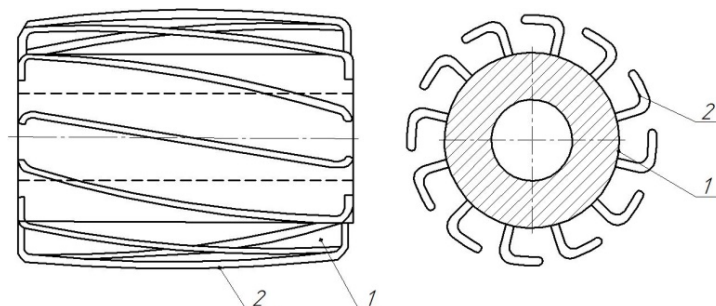
Рисунок. 3. Висівний апарат: 1 - барабан, 2 - скоби.
