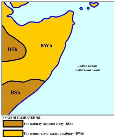
Рис. 49. Кліматі регіону півострова Сомалі (Beck et al. 2018; Холявчук 2019)
