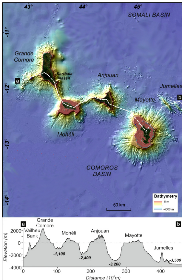
Рис. 89. Вулканічні споруди Коморських островів та їхній гіпсометричний профіль (Tzevahirtzian et al. 2021)
