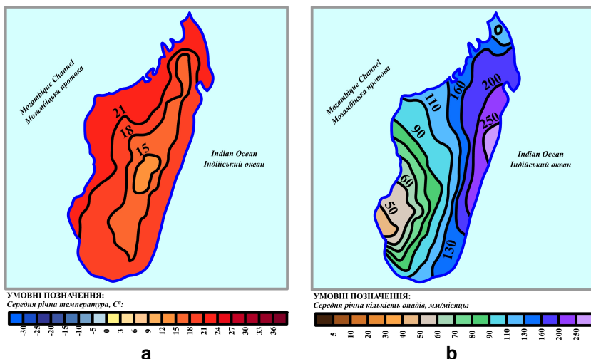
Рис. 84. Розподіл середніх річних температур (а) та середньої річної кількості опадів (b) на Мадагаскарі (1961–1990) (New et al. 1999)
