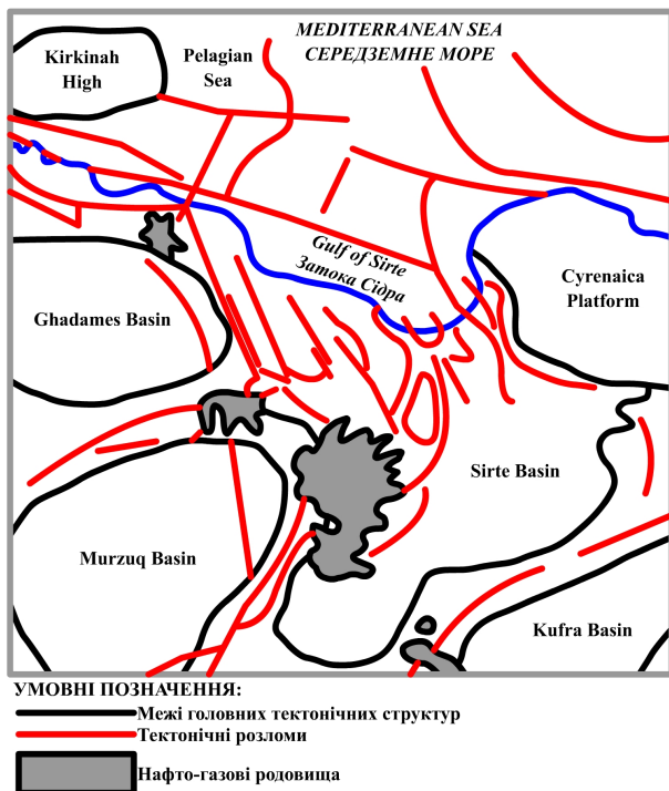
Рис. 7. Розломи басейна Сірт (Tawadros 2011)
