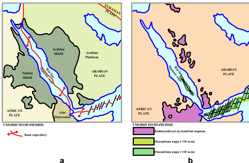
Рис. 36. Основні тектонічні структури регіону Червоного моря й Аденської затоки (а) та тектонічні особливості Великої рифтової системи Червоного моря та Аденської затоки (b) (Rasul, Stewart 2015)
