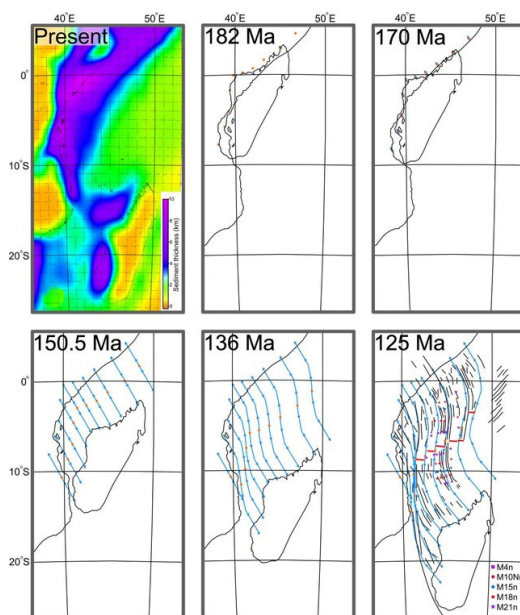
Рис. 82. Тектонічна реконструкція рифтингу Мадагаскару від Африки починаючи з раннього юрського періоду (Phethean et al. 2016)
