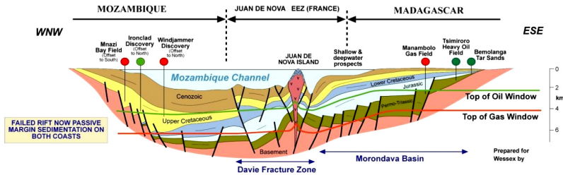
Рис. 43. Схематичний геологічний профіль через Мозамбіцьку протоку (Roberts et al. 2013)
