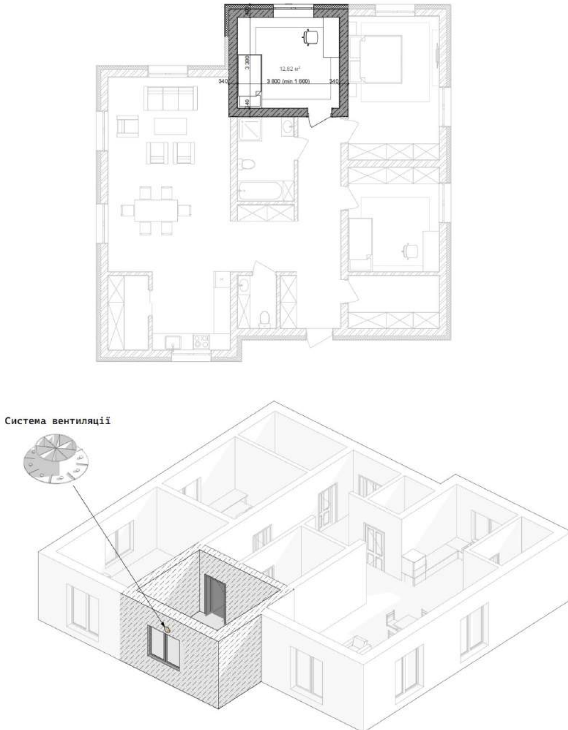
Рис. 1- План та 3-Д зображення захищеної кімнати – мамад у структурі житлового одноквартирного будинку
