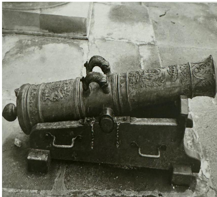
Трифунтова гармата зразка 1753 року з гербом гетьмана Кирила Розумовського.
