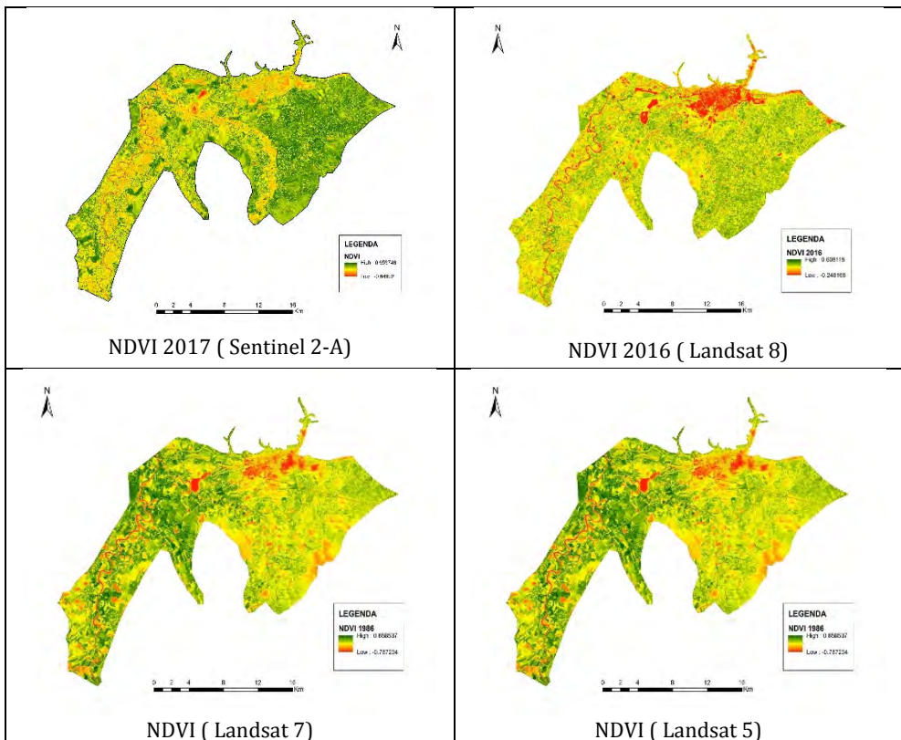
Fig 7. NDVI
